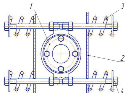
Рисунок 3 – Пружинный блок
